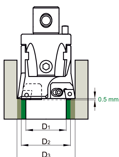
Cartuccia sfalsata
