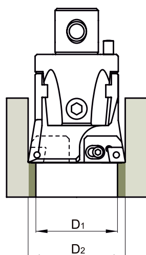
Cartuccia simmetrica
